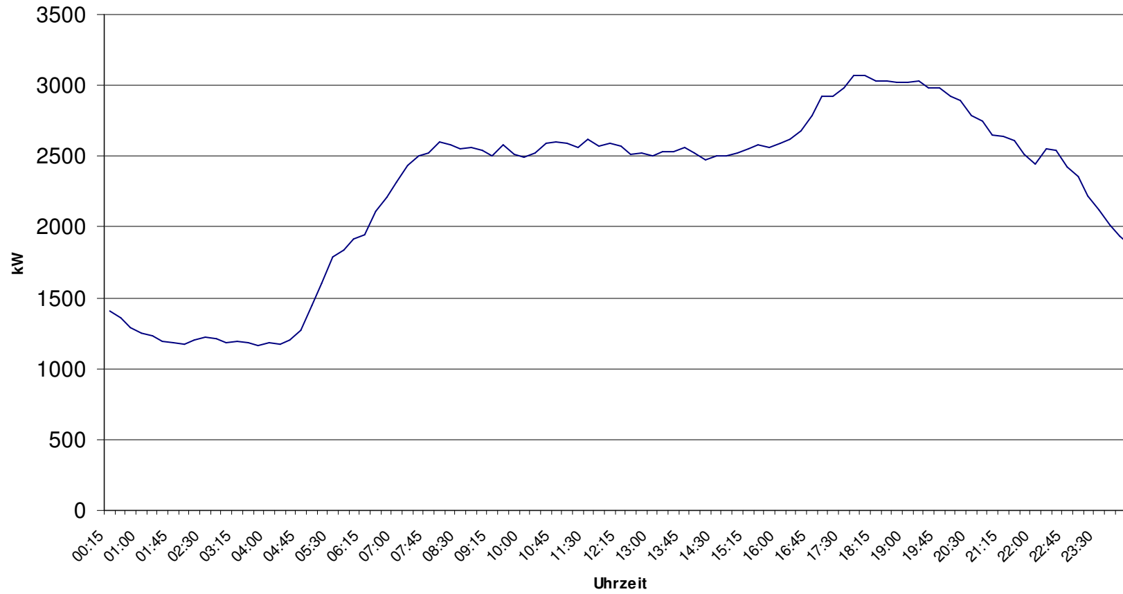
Lastverlauf am Tag der Netzhöchstlast 2005
